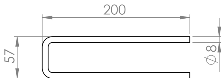
LKS.ES.8.200.G
