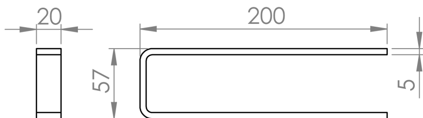
LKS.ES.20x5.200.G
